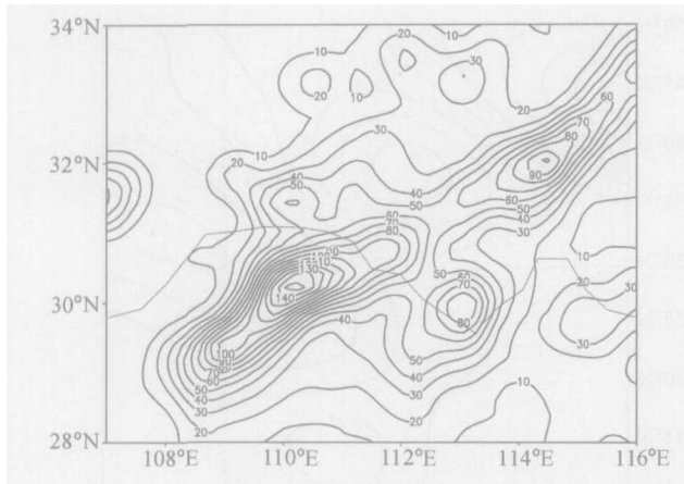
图 14 DIRA TOVS 试验区域 D01 模拟的 7 月 22 日 0000 UTC ~ 23 日 0000 UTC 24 h 降雨分布(单位: mm)
