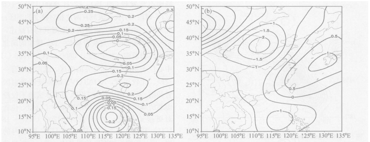
图 12 7 月 22 日 0000 UTC (a) 500 hPa、(b) 850 hPa 比湿增量场(单位: g \cdot kg^{-1} )
