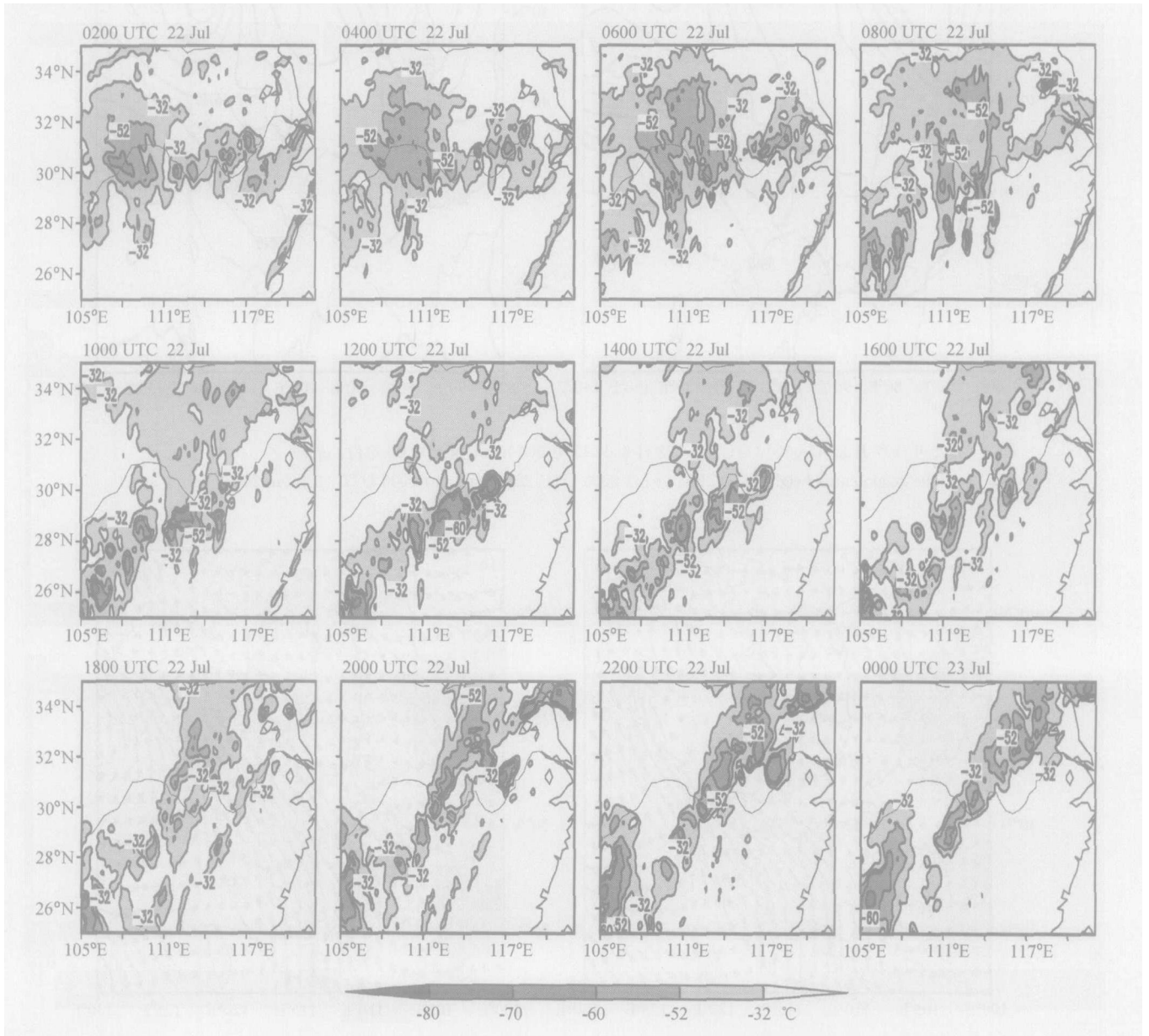
图 5 2002 年 7 月 22 日 0200 UTC ~ 23 日 0000 UTC TBB 分布
