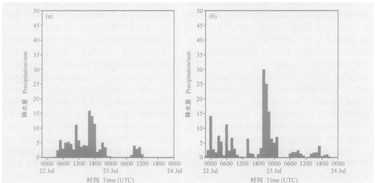
图 2 2002 年 22 日 0000 UTC~24 日 0000 UTC 逐时降雨量分布: (a) 五峰; (b) 石门
