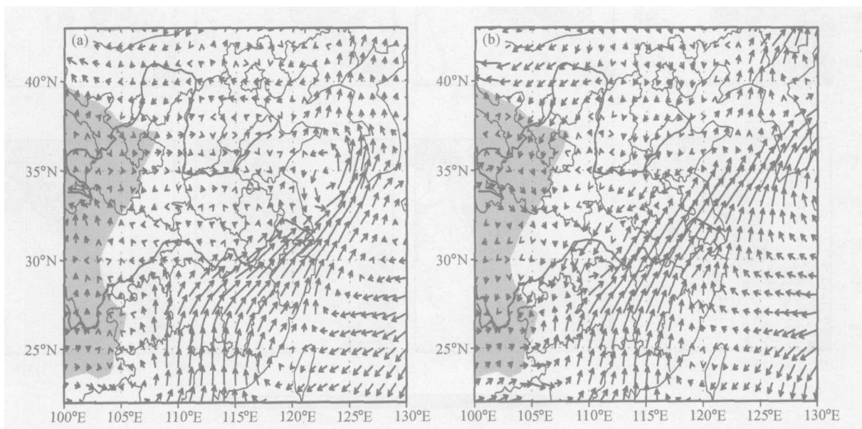
图 4 2002 年(a)7 月 22 日 0000 UTC、(b) 23 日 0000 UTC 850 hPa 风场(单位: m \cdot s^{-1} , 阴影: 地形 > 1500 m)
