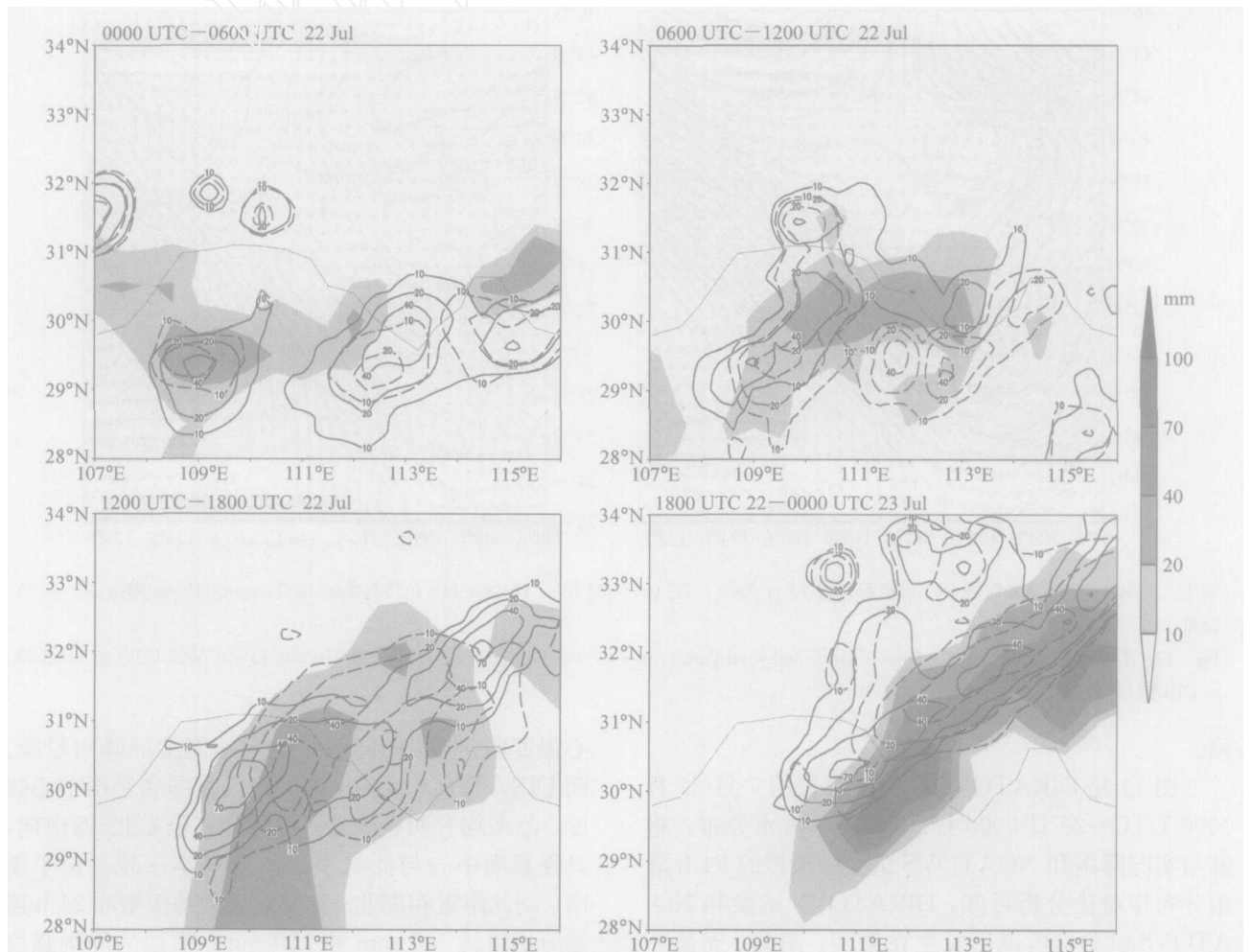
图 15 2002 年 7 月 22 日 0000 UTC ~ 23 日 0000 UTC 每 6 h 实况降雨(阴影)与 DIRA TOVS(实线)、NOA TOVS(虚线) 试验区域 D01 模拟的每 6 h 降雨分布(单位: mm)
