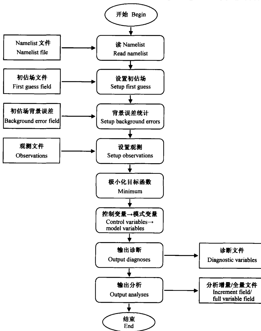
图 6 三维变分同化系统程序流程
