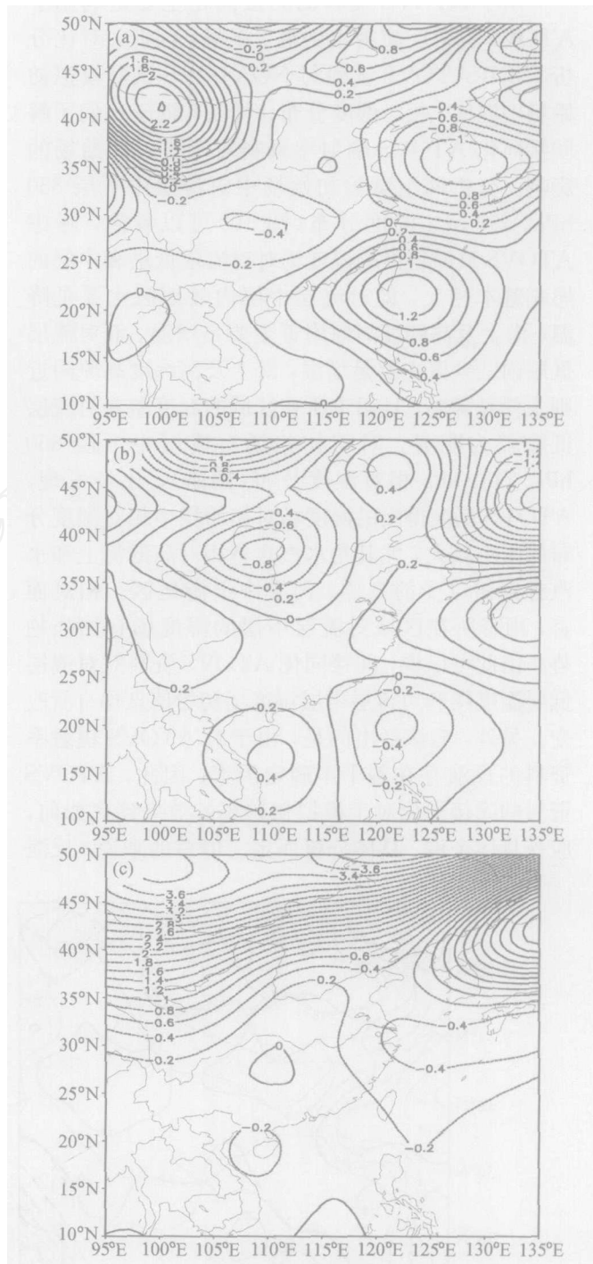
图 11 7 月 22 日 0000 UTC (a) 300 hPa、(b) 500 hPa、(c) 850 hPa 温度增量场(单位: )
