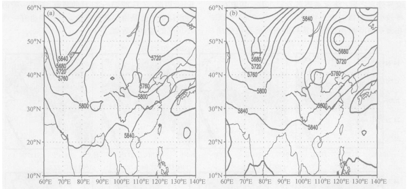
图 3 2002 年(a)7 月 22 日 0000 UTC、(b) 23 日 0000 UTC 500 hPa 位势高度场(单位: gpm)
