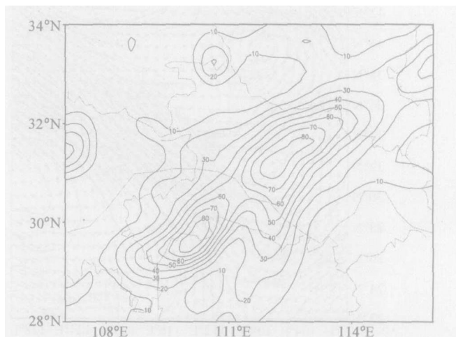
图 9 INDIRA TOVS 试验区域 D01 模拟的 7 月 22 日 0000 UTC~23 日 0000 UTC 24 h 降雨分布(单位: mm)
