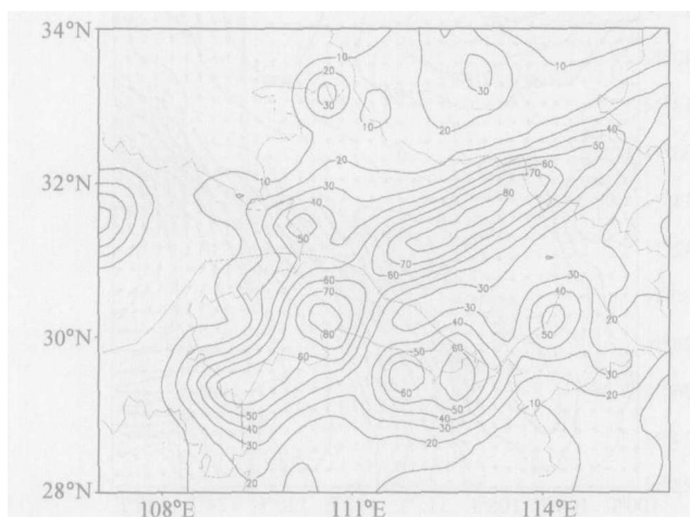
图 8 NOATOVS 试验区域 D01 模拟的 7 月 22 日 0000 UTC~23 日 0000 UTC 24 h 降雨分布(单位: mm)
