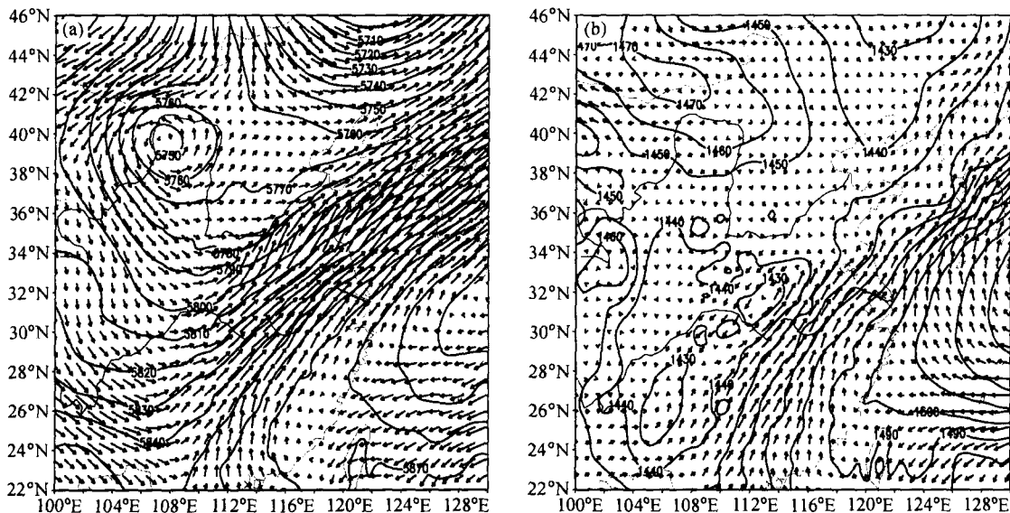
图 7 NOATOVS 试验区域 D01 模拟的 7 月 23 日 0000 UTC 位势高度场(单位: gpm)与风场(单位: m \cdot s^{-1} )分布: (a) 500 hPa; (b) 850 hPa
