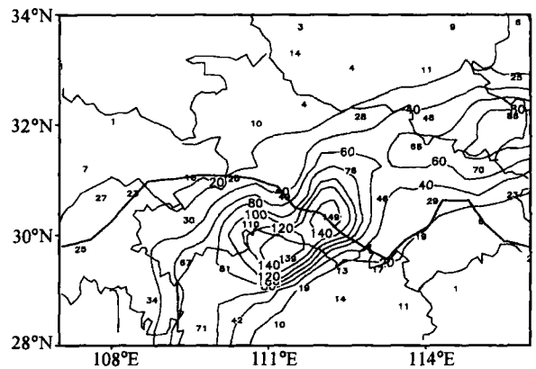
图 1 2002 年 7 月 22 日 0000 UTC~23 日 0000 UTC 24 h 实况降雨分布(单位: mm)
