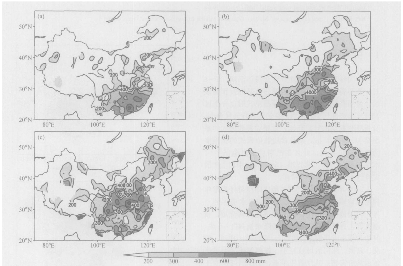
图2 2005年5~8月的月降雨量: (a) 5月; (b) 6月; (c) 7月和 (d) 8月
