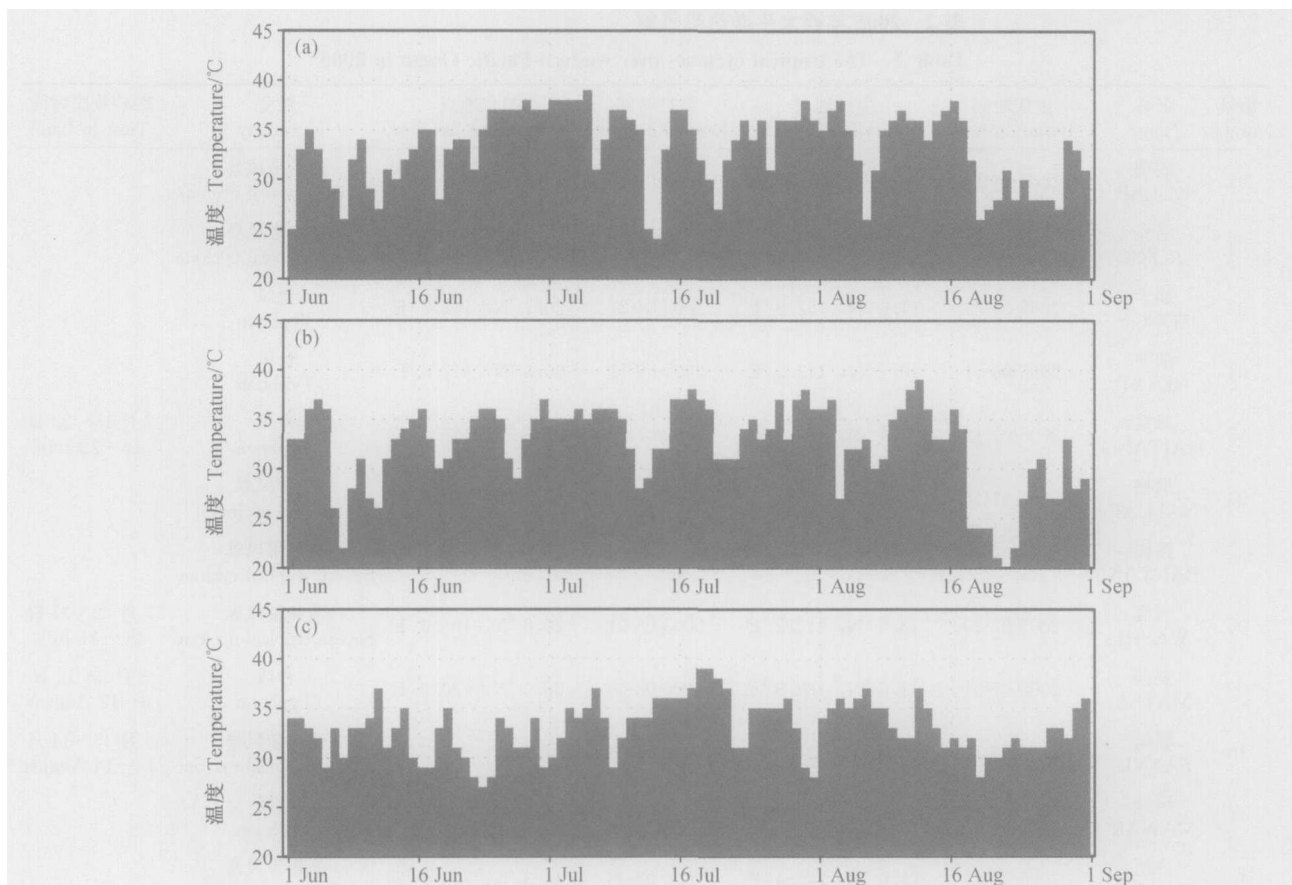
图 14 2005 年 6~8 月杭州 (a)、武汉 (b) 和广州 (c) 的日最高气温分布
