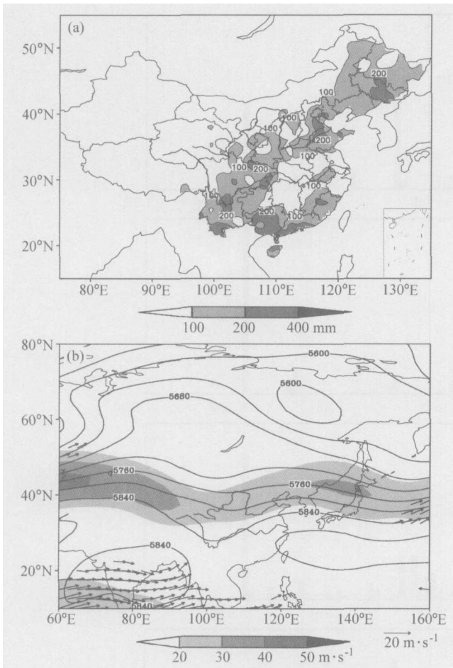
图 8 1994 年梅雨期 (6 月 18 日~7 月 10 日) 的降雨量 (a) 和环流 (b)。 (b) 中: 阴影为 200 hPa 风速 > 20 \text{ m} \cdot \text{s}^{-1} , 风矢量为 850 hPa 上风速 > 8 \text{ m} \cdot \text{s}^{-1} , 等值线为 500 hPa 位势高度场 (单位: gpm)
