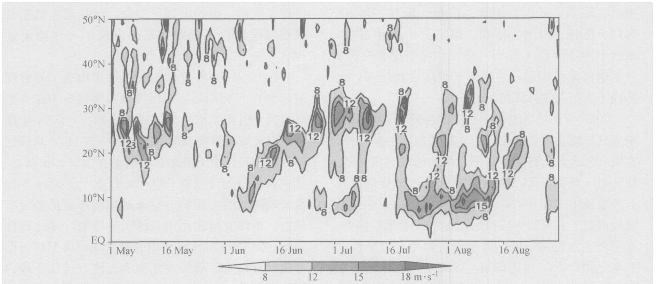
图 3 2005 年 5 月 1 日 ~ 8 月 31 日 110 ~ 120 度的平均风速
