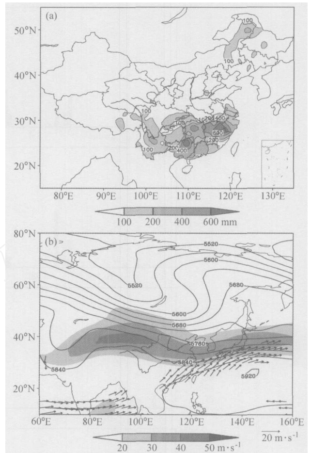
图 9 1998 年第 1 阶段梅雨期 (6 月 12 ~ 28 日) 的降雨量 (a) 和环流 (b)。 (b) 中: 阴影为 200 hPa 风速 > 20 \text{ m} \cdot \text{s}^{-1} , 风矢量为 850 hPa 上风速 > 8 \text{ m} \cdot \text{s}^{-1} , 等值线为 500 hPa 位势高度场 (单位: gpm)
