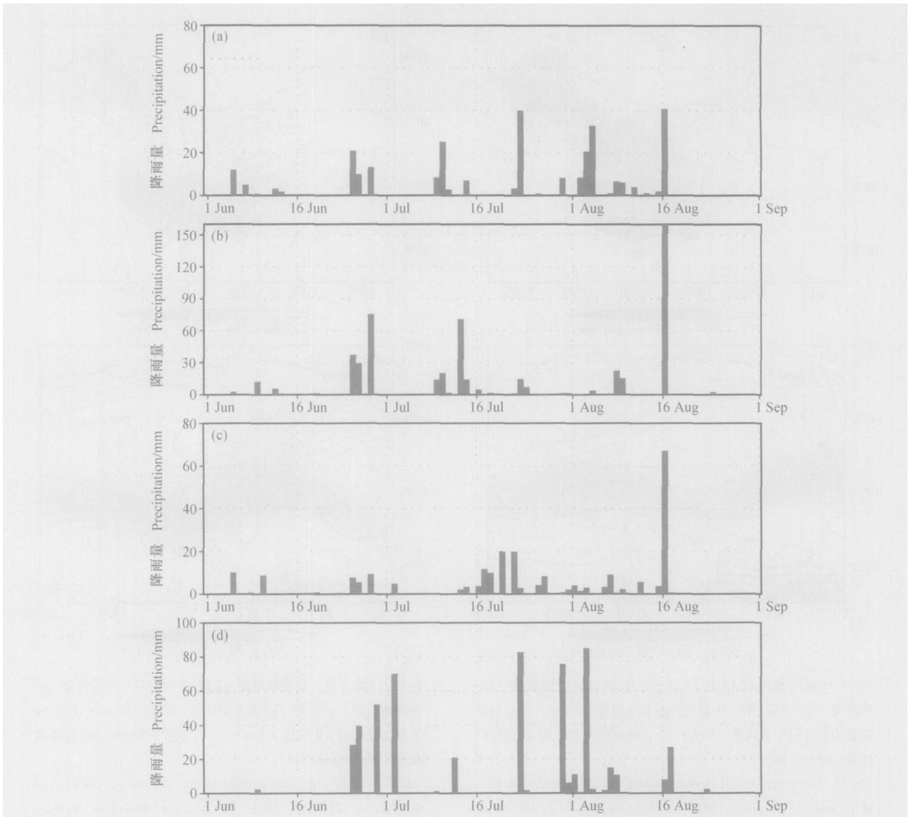
图 10 2005 年 6~8 月逐日降雨量: (a) 北京; (b) 天津; (c) 石家庄; (d) 济南
