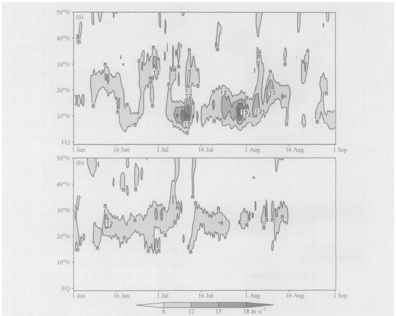
图7 1994 (a) 和 1998 (b) 6~8月 110~120 hPa 平均风速
