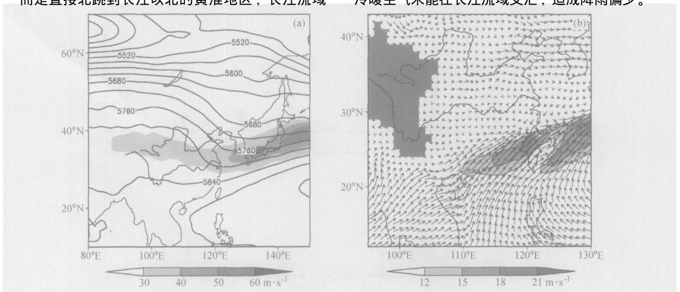
图 5 2005 年 6 月 17~23 日的平均环流: (a) 500 hPa 位势高度(等值线, 单位: gpm) 和 200 hPa 的风速(阴影为风速 > 30 \text{ m} \cdot \text{s}^{-1} ); (b) 850 hPa 风场(浅阴影为风速 > 12 \text{ m} \cdot \text{s}^{-1} , 左侧深色阴影为地形高于 1 500 m)
