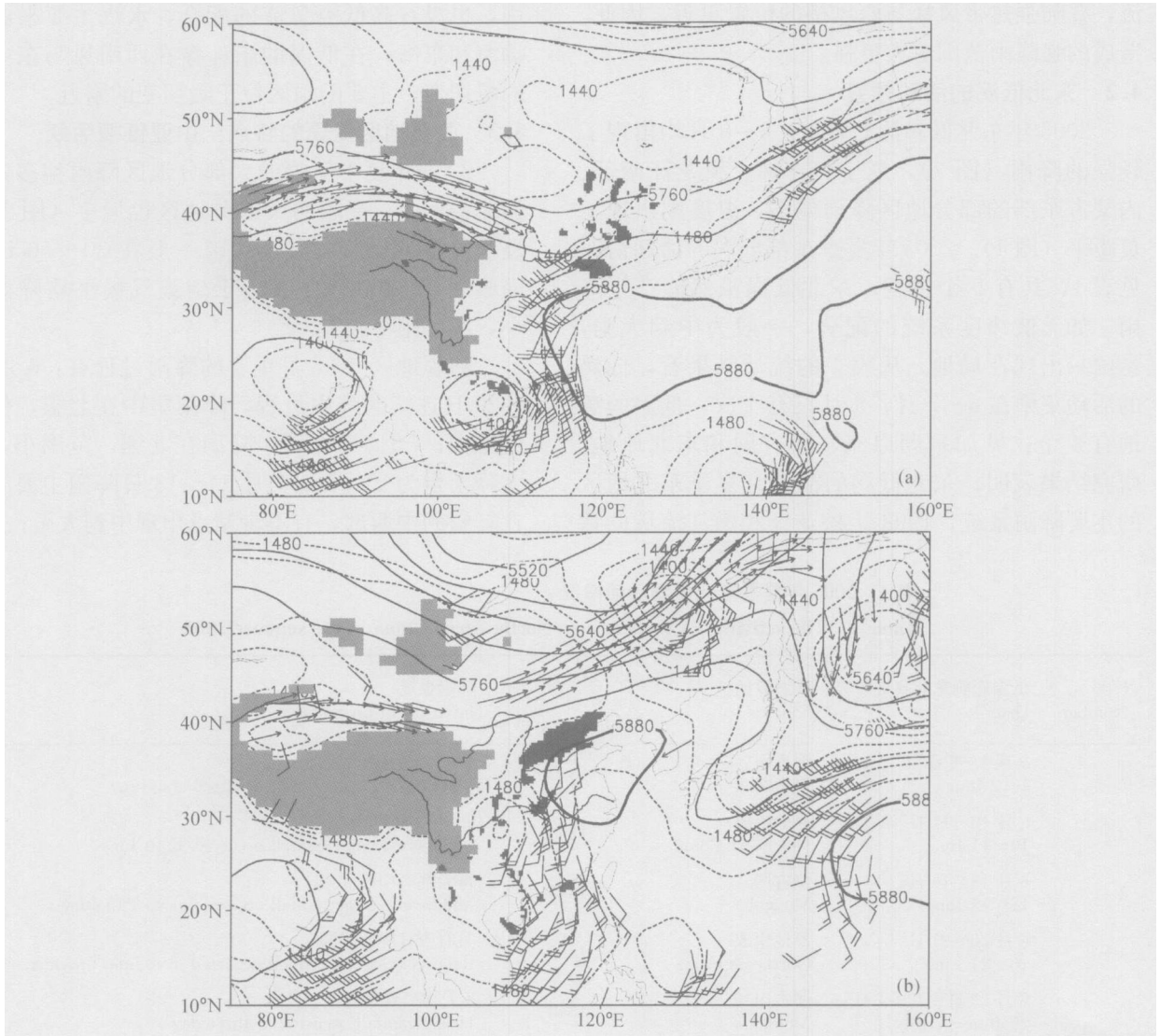
图 11 2005 年 7 月 31 日 (a) 和 8 月 16 日 (b) 天气形势合成。浅色阴影区为地形 > 1 500 m；深色阴影区表示 24 h 降雨量 > 25 mm 的强降雨中心；箭矢线为 200 hPa 上风速 > 40 m · s -1 的高空急流，风标为 850 hPa 上风速 > 8 m · s -1 的低空急流；粗实线和虚线分别为 500 hPa 和 850 hPa 等高线（单位：gpm）
