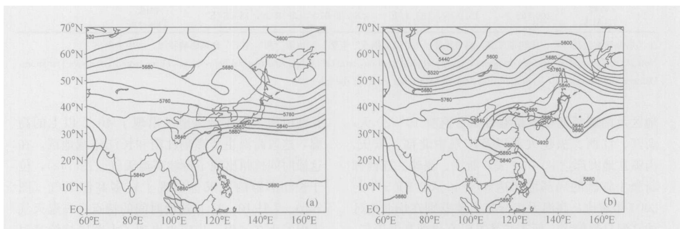
图 15 2005 年 6 月 26 日~7 月 8 日 (a) 和 8 月 11~12 日 (b) 的 500 hPa 平均高度场 (单位: gpm)
