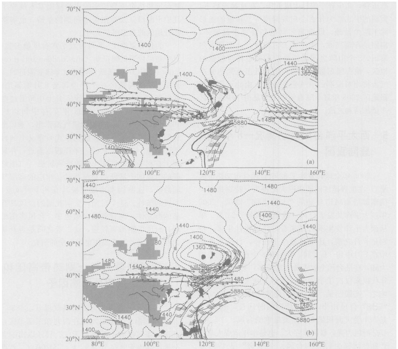
图 12 2005 年 6 月 29 日 (a) 和 30 日 (b) 天气形势合成。浅色阴影区为地形高于 1 500 m；深色阴影区表示 24 h 降雨量 > 10 mm 的强降雨中心；箭矢线为 200 hPa 上风速 > 40 m · s -1 的高空急流，风标为 850 hPa 上风速 > 12 m · s -1 的低空急流；粗实线和虚线分别为 500 hPa 和 850 hPa 等高线（单位：gpm）
