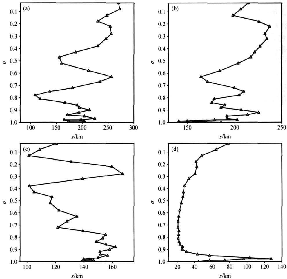
图3 同图2，但为 15 km 模拟区域的长度尺度 Fig. 3 The same as Fig. 2, but for length scale of 15 km domain
