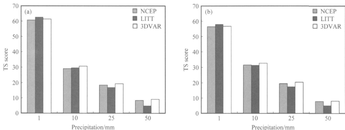
图 6 2005 年 8 月 1~31 日试验月平均的降雨量 TS 评分: (a) 区域 1 (45 km); (b) 区域 2 (15 km)
