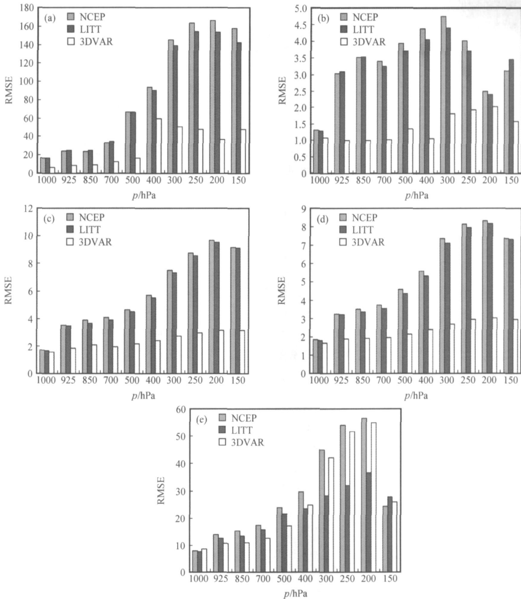
图 7 3 个试验形势场的 24 h 预报结果与站点探空的均方根误差分布: (a) 高度场 (单位: gpm); (b) 温度场 (单位: °C); (c) 纬向风 (单位: m · s -1 ); (d) 经向风 (单位: m · s -1 ); (e) 相对湿度 (%)
