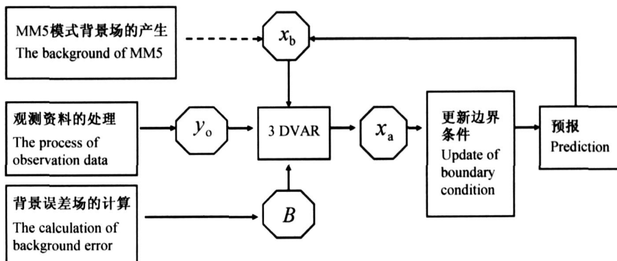
图 1 MM5/3DVAR 的流程及其与 MM5 模式的关系
