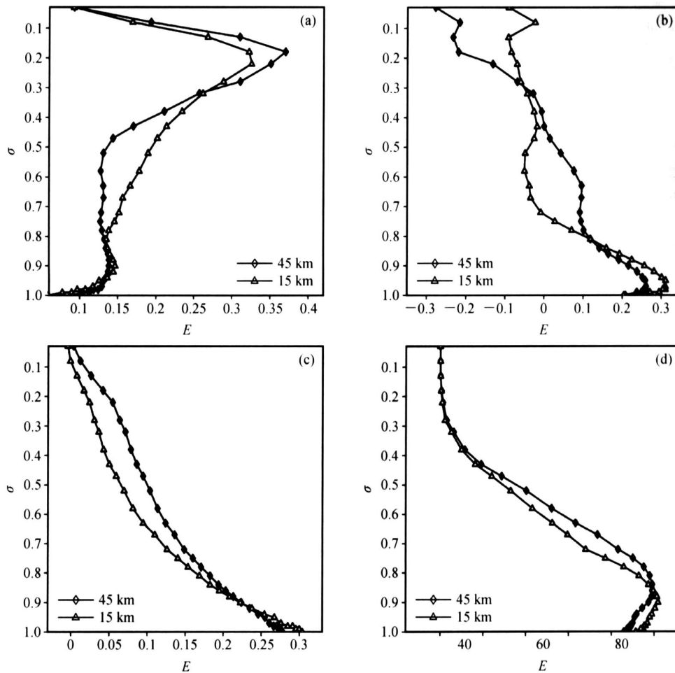
图5 模拟区域1和2的背景误差协方差矩阵的区域平均第1特征向量 E : (a) 流函数; (b) 速度势; (c) 非平衡气压; (d) 比湿 Fig. 5 The first eigenvector of the vertical component of domain-averaged background error covariance matrix for (a) stream function, (b) velocity potential, (c) unbalance pressure, and (d) specific humidity
