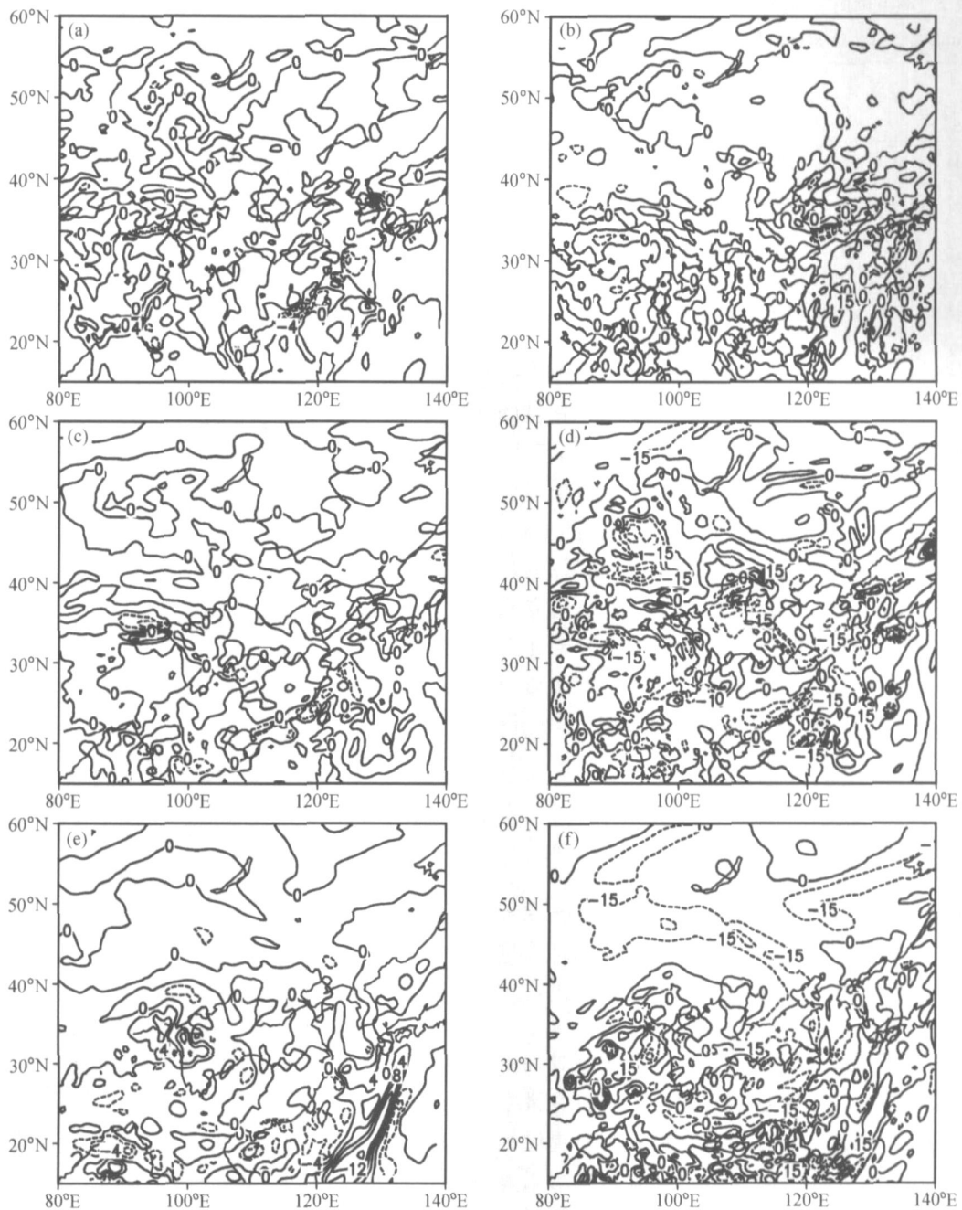
图9 2005年8月19日的24 h 预报风场(左侧, 单位: m \cdot s^{-1} )和相对湿度场(右侧, % ) 3DVAR 试验与LITT 试验的差值: (a)、(b) 850 hPa; (c)、(d) 500 hPa; (e)、(f) 200 hPa
