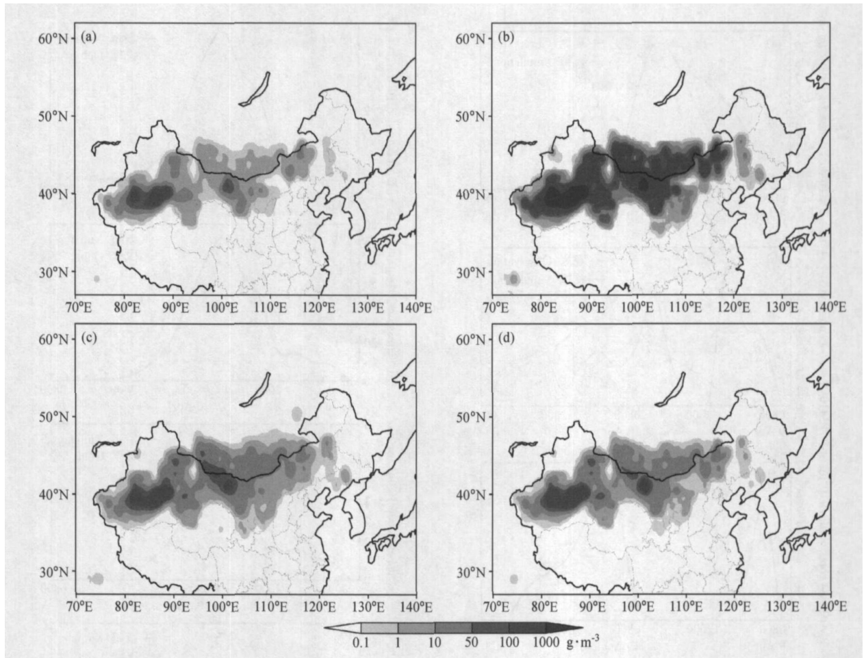
图 8 模拟的 2006 年 4 月 9 日 8 时~11 日 8 时的总起沙量: (a) d < 2 \mu\text{m} ; (b) 2 \mu\text{m} < d < 11 \mu\text{m} ; (c) 11 \mu\text{m} < d < 22 \mu\text{m} (c) 总和 Fig. 8 The simulated dust emission for different particle size group form 0800 LST 9 Apr to 0800 LST 11 Apr 2006: (a) d < 2 \mu\text{m} ; (b) 2 \mu\text{m} < d < 11 \mu\text{m} ; (c) 11 \mu\text{m} < d < 22 \mu\text{m} ; (d) total
