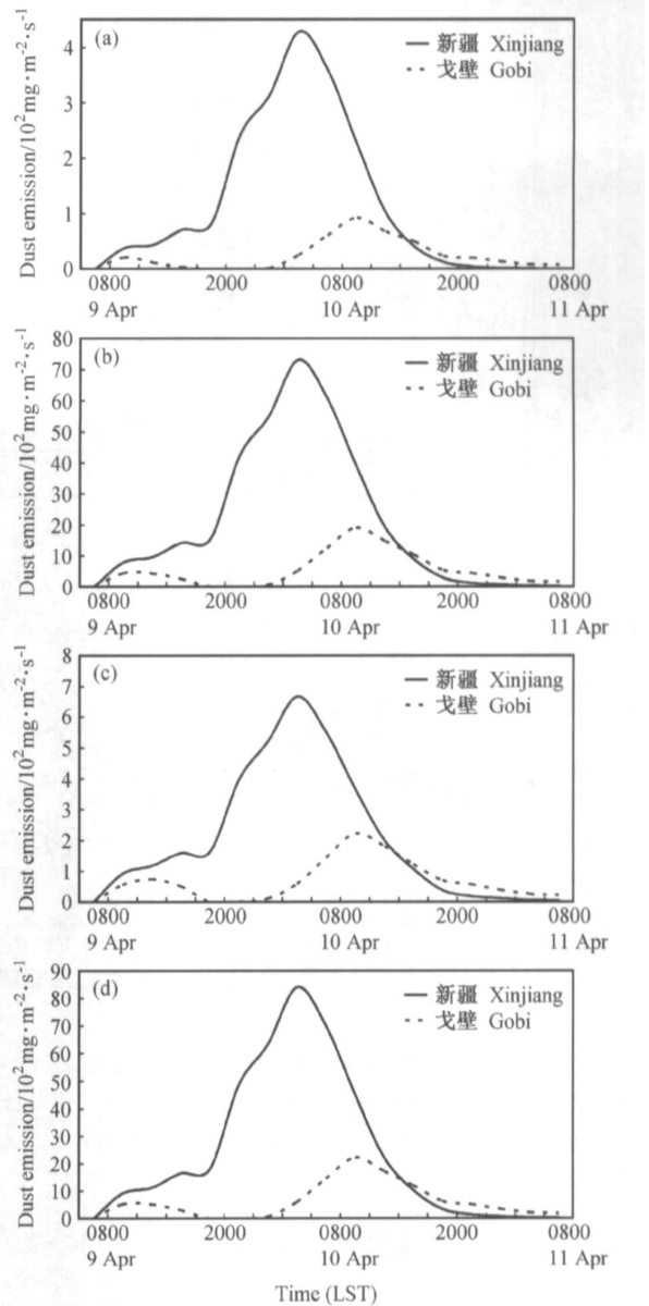
图7 2006年4月9日8时~11日8时新疆地区和戈壁地区不同粒径 (d) 沙尘起沙量随时间演变：(a) d < 2 \mu\text{m} ；(b) 2 \mu\text{m} < d < 11 \mu\text{m} ；(c) 11 \mu\text{m} < d < 22 \mu\text{m} ；(d) 各粒径之和
