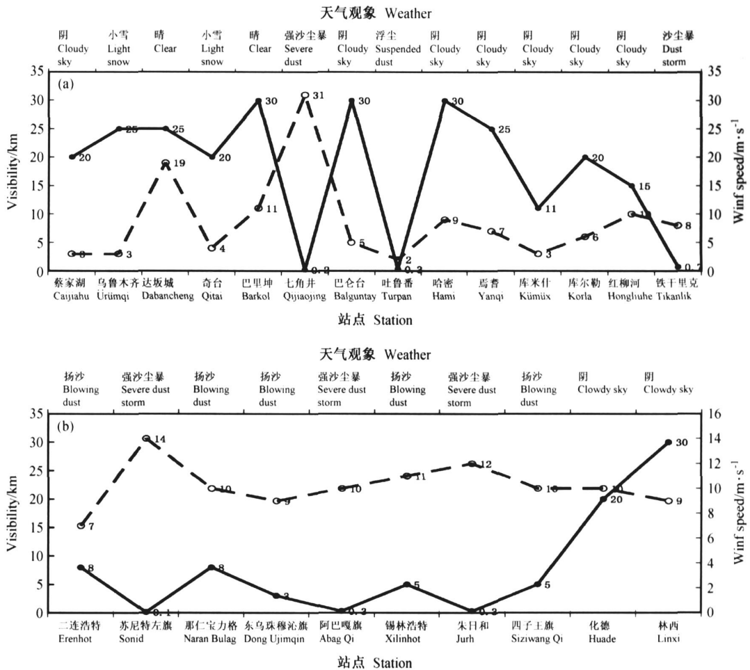
图3 2006年4月强沙尘暴过程新疆地区和内蒙古地区的能见度、风速和天气现象 (a) 新疆东部地区4月10日8时; (b) 内蒙古中东部4月10日14时
