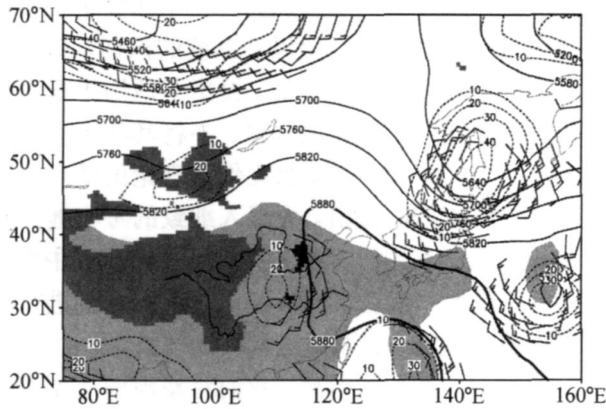
图2 1996年8月4日登陆台风北上受高压阻挡停滞天气形势合成分布(引自文献[70])。浅阴影: 850 hPa \theta_{se} \geq 338 K; 深阴影: 地形大于1500 m; 黑色阴影: 24 h 降雨量 \geq 50 mm 的暴雨中心。风标: 风速 \geq 12 m/s 表示 850 hPa 上的低空急流; 粗实线: 500 hPa 等高线(单位: gpm); 短虚线: 500 hPa 上的等涡度线(单位: 10^{-5} s^{-1} )
