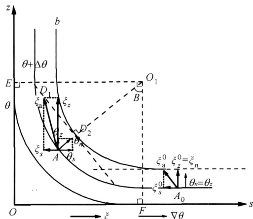
图 1 上滑情况下的倾斜涡度发展示意图 (引自文献 [19]) Fig. 1 Schematic diagram of up-sliding slantwise vorticity development (from reference [19])
