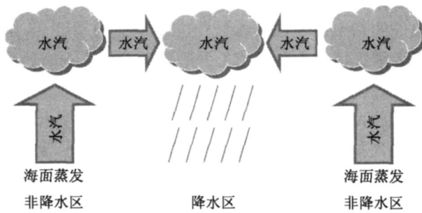
图4 海面蒸发在地面降水过程中作用示意图
