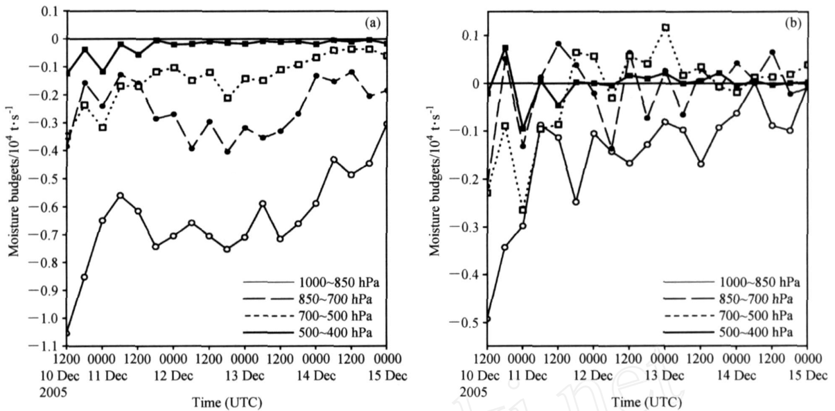
图 13 2005 年 12 月 10~15 日 1 000~850、850~700、700~500 和 500~400 hPa 4 个层次水汽收支随时间的变化：(a) 北边界；(b) 北边界 - 南边界（以向北方向为正值，单位： 10^4 t \cdot s^{-1} ）
