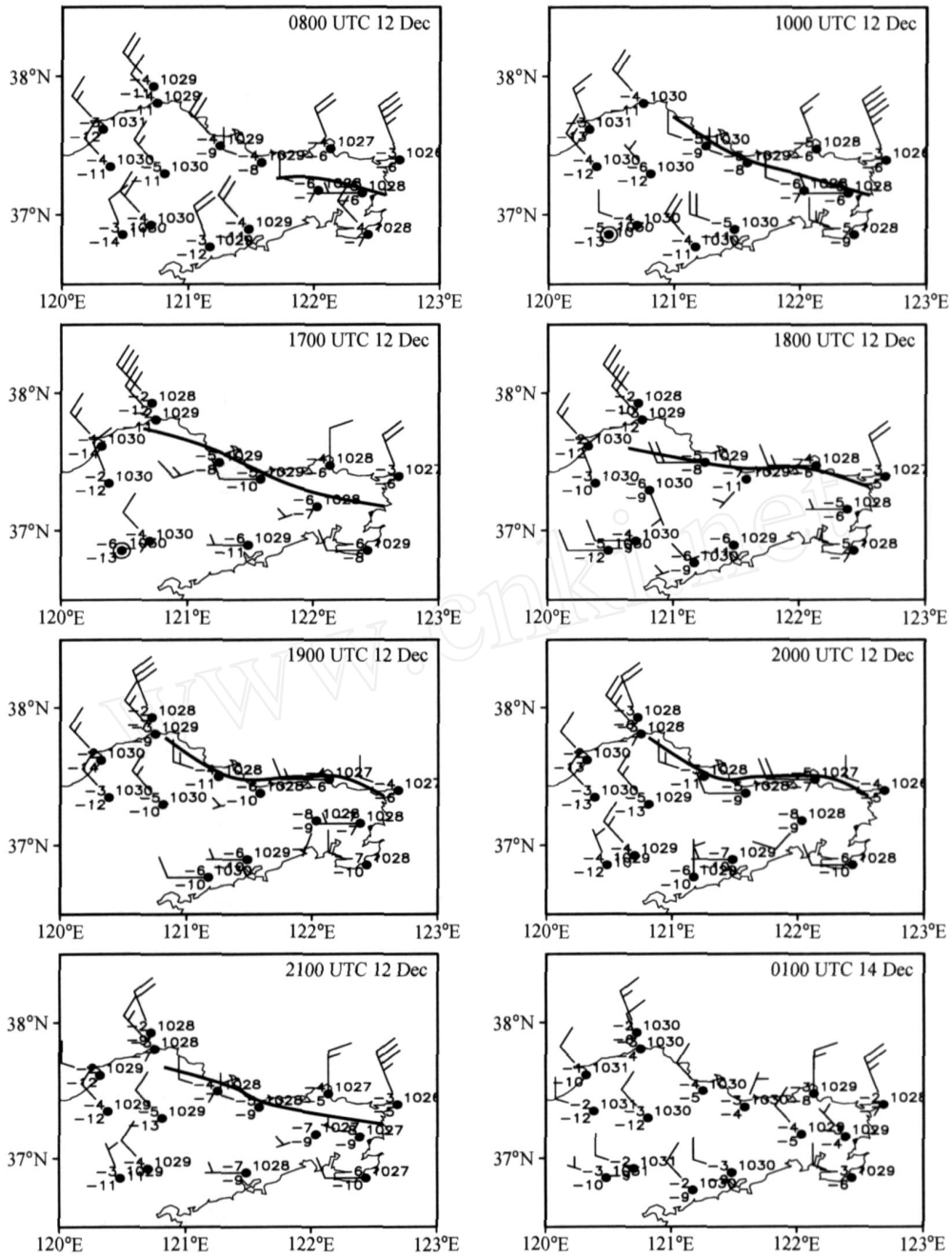
图7 同图6, 但为12日8时~14日1时
