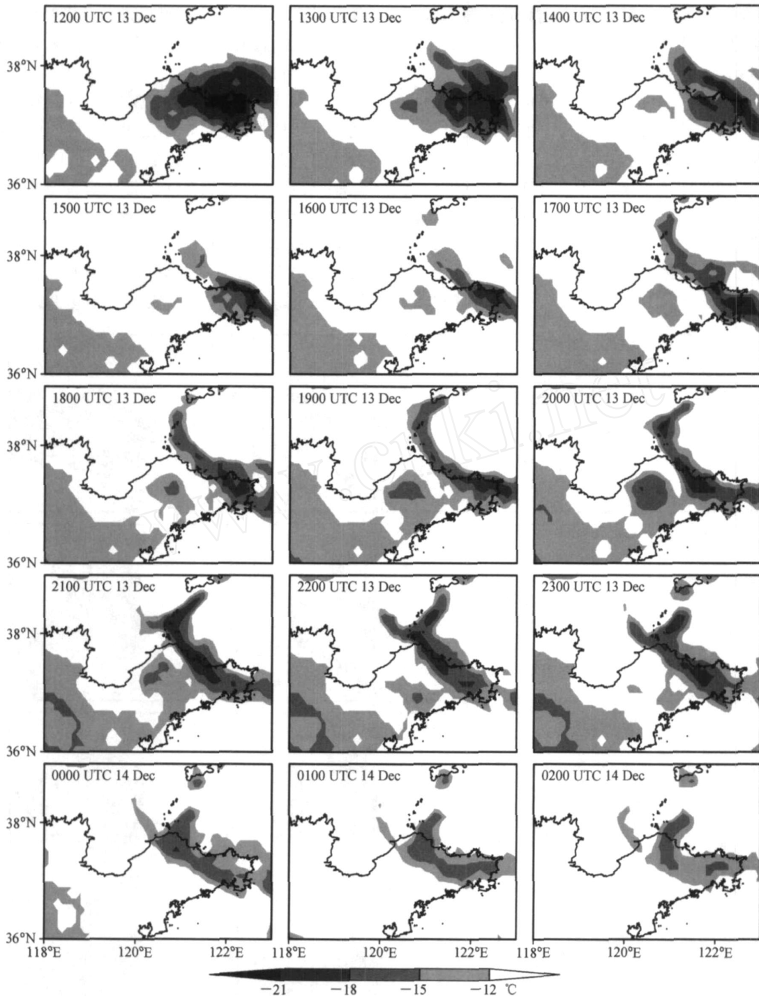
图 10 2005 年 12 月 13 日 12 时~14 日 2 时 TBB 分布
