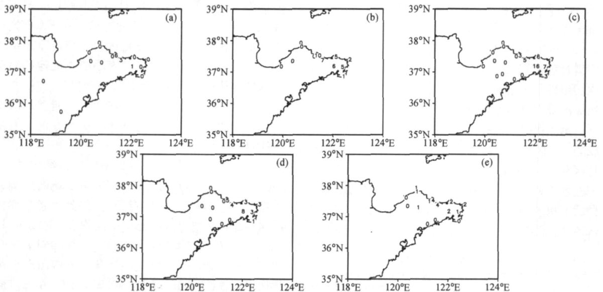
图 2 2005 年 12 月 10~15 日 24 h 降水量 (单位: mm): (a) 10 日 0 时~11 日 0 时; (b) 11 日 0 时~12 日 0 时; (c) 12 日 0 时~13 日 0 时; (d) 13 日 0 时~14 日 0 时; (e) 14 日 0 时~15 日 0 时
