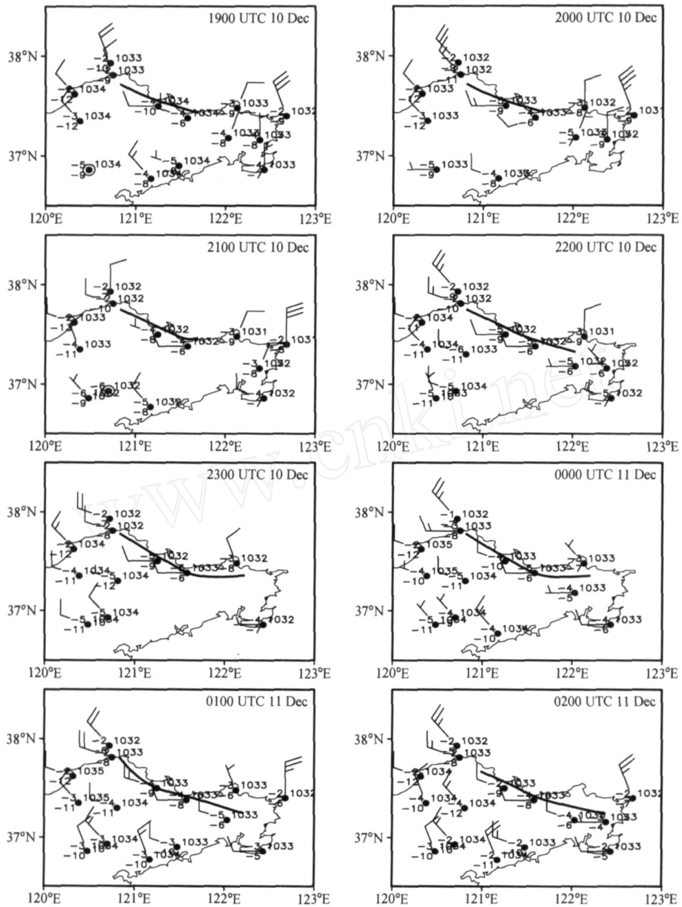
图6 2005年12月10日19时~11日2时自动观测站点气象要素的分布(温度、露点单位: ^{\circ}\text{C} , 地面气压单位: hPa, 风速单位: \text{m}\cdot\text{s}^{-1} , 粗实线为海岸锋)
