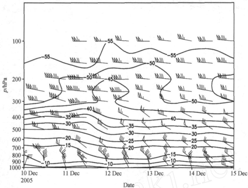
图4 2005年12月10日0时~15日0时成山头(54776)探空站的风场(风羽:满杆和半杆分别为4和2 \text{m} \cdot \text{s}^{-1} , 旗子为20 \text{m} \cdot \text{s}^{-1} )和温度(实线, 单位: ^{\circ}\text{C} )的时间-高度变化
