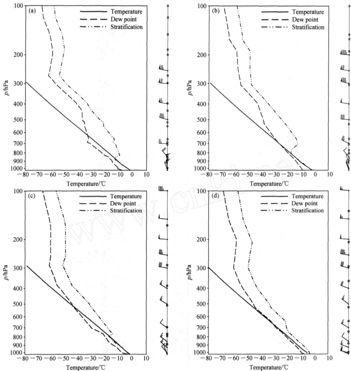
图5 2005年12月成山头探空曲线：(a) 10日12时；(b) 11日0时；(c) 14日12时；(d) 15日0时
