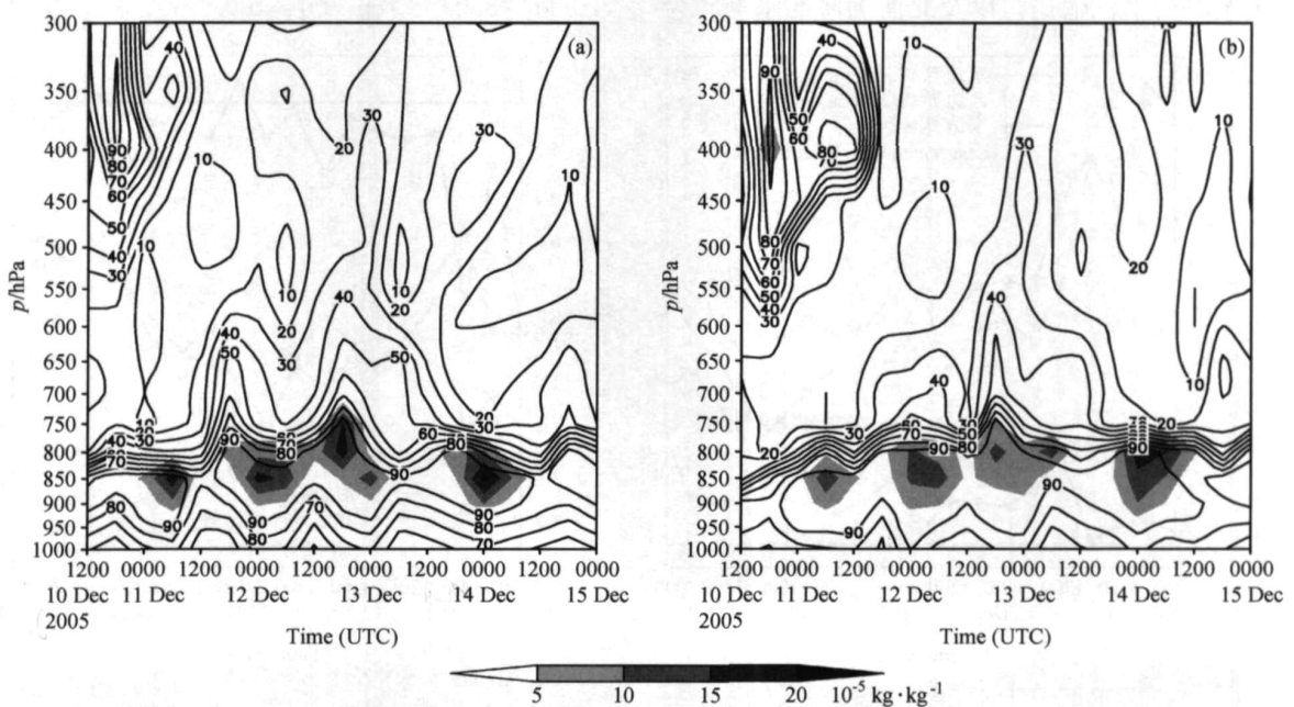
图 11 云水含量 (阴影) 和相对湿度 (实等值线, %) 的时间-高度变化: (a) (38°N, 121°E); (b) (37°N, 122°E)
