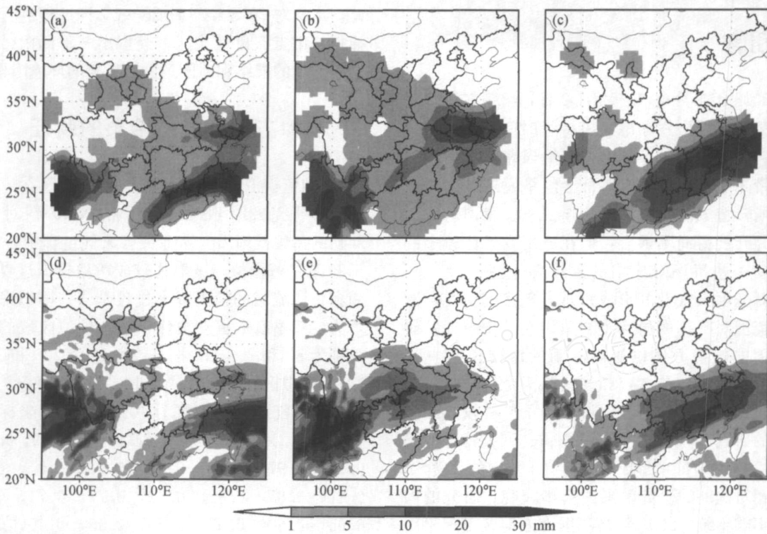
图1 2008年1月26~28日模拟(上行)和观测(下行)的24 h降水量。(a)、(d) 26日0000 UTC~27日0000 UTC, (b)、(e) 27日0000 UTC~28日0000 UTC, (c)、(f) 28日0000 UTC~29日0000 UTC
