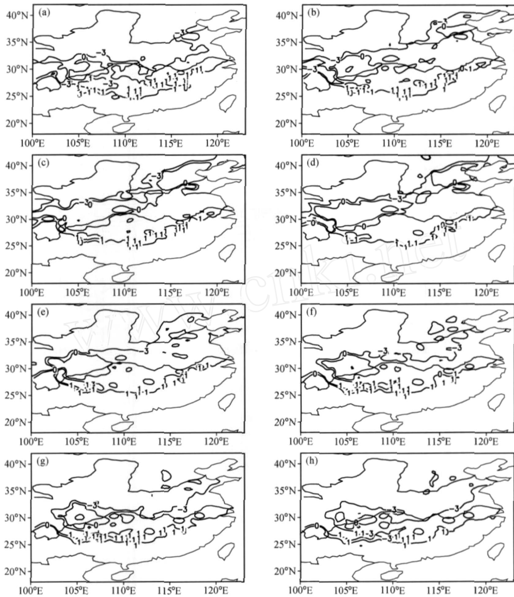
图 4 2008 年 1 月 28 日的地面温度 (实线, 单位: ^{\circ}\text{C} ) 和冻雨分布 (数字 1): (a) 0000 UTC, (b) 0300 UTC, (c) 0600 UTC, (d) 0900 UTC, (e) 1200 UTC, (f) 1500 UTC, (g) 1800 UTC, (h) 2100 UTC Fig 4 The surface temperature (solid line, units: ^{\circ}\text{C} ) and freezing rain (number 1) on 28 Jan 2008: (a) 0000 UTC, (b) 0300 UTC, (c) 0600 UTC, (d) 0900 UTC, (e) 1200 UTC, (f) 1500 UTC, (g) 1800 UTC, (h) 2100 UTC
