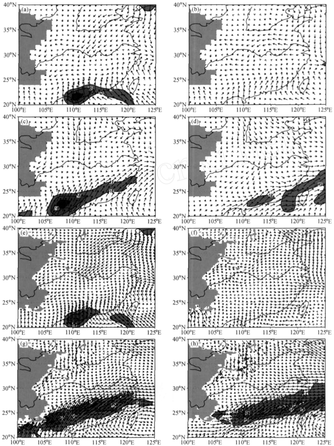
图 2 2008 年 1 月 26 ~ 29 日观测 (a) ~ (d) 和模拟 (e) ~ (h) 的 850 hPa 风场。深色阴影为低空急流 ( 12 \text{ m} \cdot \text{s}^{-1} ), 浅色阴影为地形大于 1 500 m。(a)、(e) 26 日 0000 UTC, (b)、(f) 27 日 0000 UTC, (c)、(g) 28 日 0000 UTC, (d)、(h) 29 日 0000 UTC
