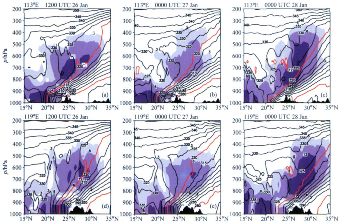
图 3 2008 年 1 月 26 ~ 28 日模拟的假相当位温 (实线, 单位: K) 和水汽通量 (阴影, 单位: \text{g} \cdot \text{s}^{-1} \cdot \text{cm}^{-1} \cdot \text{hPa}^{-1} ) 沿 113°E (上行) 和 119°E (下行) 的垂直剖面。黑色阴影为地形。(a)、(d) 26 日 1200 UTC, (b)、(e) 27 日 0000 UTC; (c)、(f) 28 日 0000 UTC
