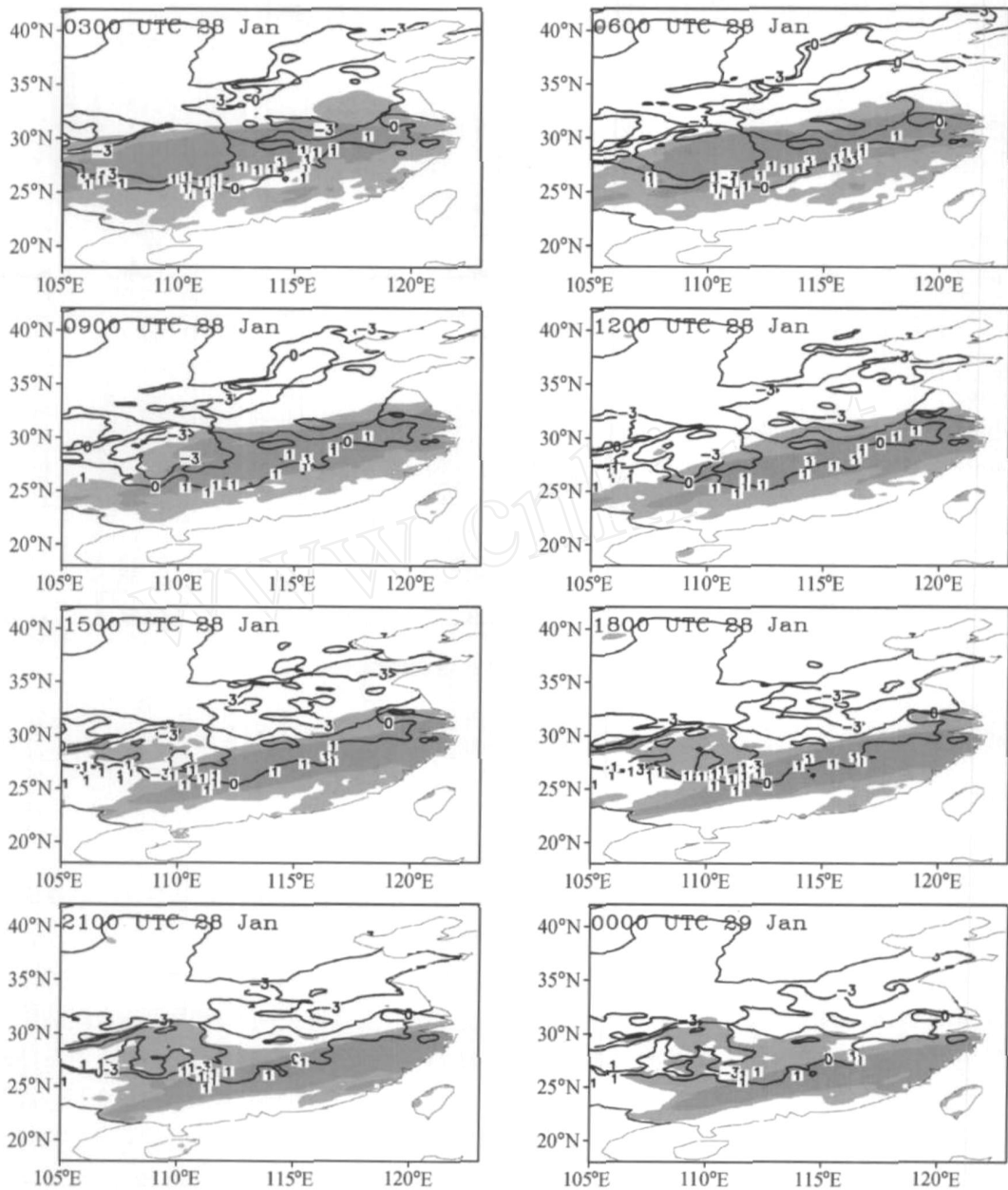
图7 2008年1月28日模拟的地面温度(实线,单位: ^{\circ}\text{C} )、3 h 降雨区(阴影)和观测的冻雨分布(数字 1)
