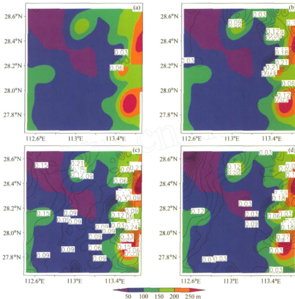
图4 2003年12月12日 (a) 13时、(b) 15时、(c) 21时、(d) 13日00时近地层液态水含量 (等值线, 单位: g \cdot kg^{-1} ) 和地形高度 (阴影) 分布图
