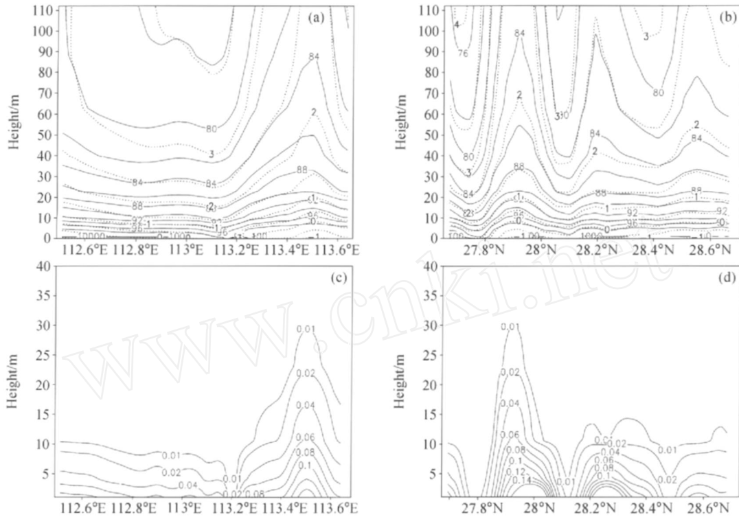
图5 2003年12月12日21时(a、b)温度(虚线,单位: )和湿度(实线,%), (c、d)液态水含量(单位: \text{g} \cdot \text{kg}^{-1} )沿(a、c) 27.9°N和(b、d) 113.5°E的垂直分布
