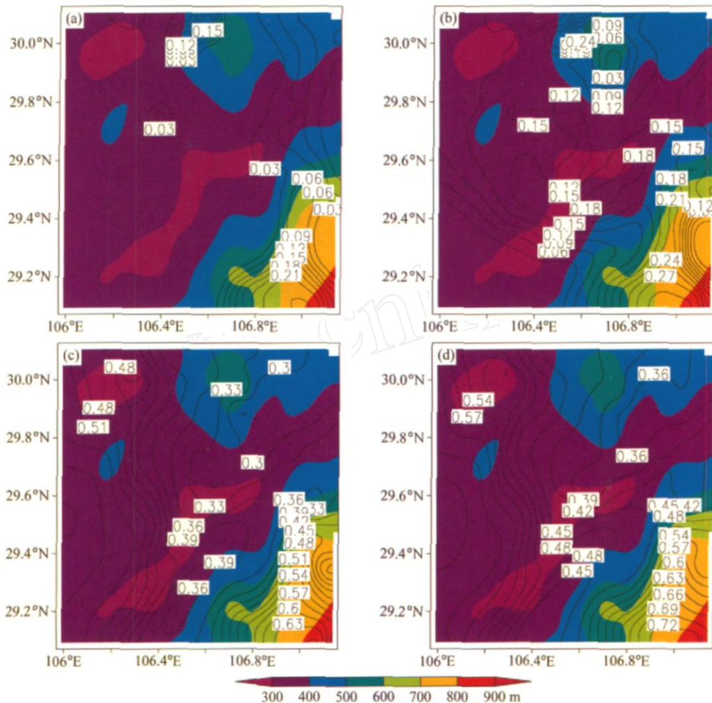
图1 2003年1月22日(a)13时30分、(b)15时、(c)21时、(d)23日00时近地层液态水含量(等值线,单位: \text{g} \cdot \text{kg}^{-1} )和地形高度(阴影)分布图
