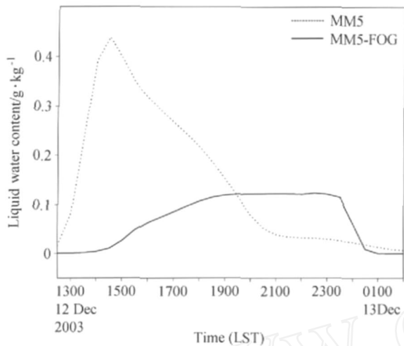
图7 MM5 和 MM5-FOG 模拟的区域平均液态水含量随时间的演变趋势
