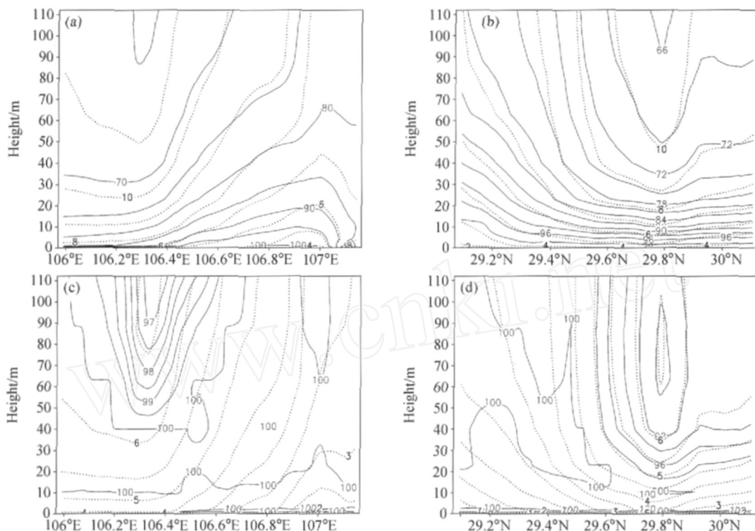
图2 2003年1月22日 (a、b) 15时和 (c、d) 21时温度 (虚线, 单位: ^{\circ}\text{C} )、湿度 (实线, %) 沿 (a、c) 29.5°N 和 (b、d) 106.5°E 垂直分布
