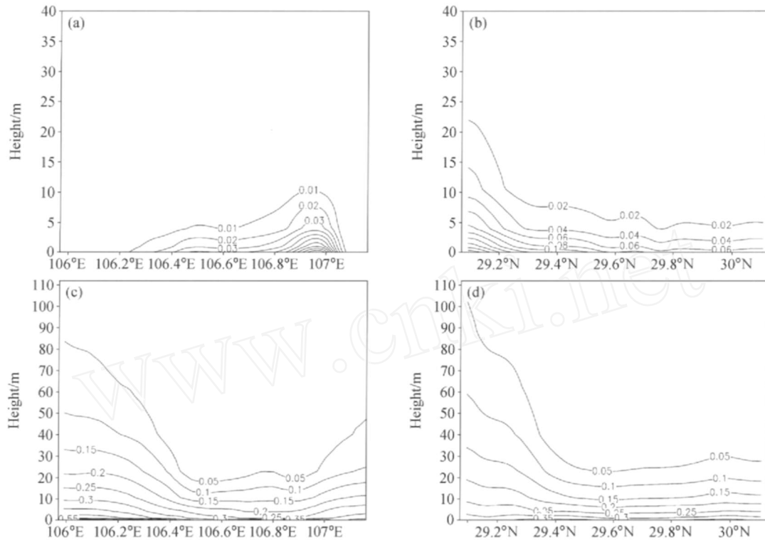
图3 2003年1月22日(a、b)15时和(c、d)21时液态水含量(单位: \text{g} \cdot \text{kg}^{-1} )沿(a、c)29.5°N和(b、d)106.5°E垂直分布 Fig. 3 The vertical cross sections for simulated liquid water content ( \text{g} \cdot \text{kg}^{-1} ) along (a, c) 29.5°N and (b, d) 106.5°E at (a, b) 1500 UTC and (c, d) 2100 UTC 22 Jan 2003
