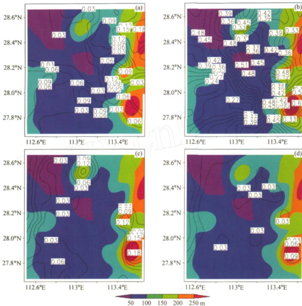
图 6 MM5 模拟的 2003 年 12 月 12 日 (a) 13 时、(b) 15 时、(c) 21 时、(d) 13 日 00 时近地层液态水含量 (等值线, 单位: g \cdot kg^{-1} ) 和地形高度 (阴影) 分布图
